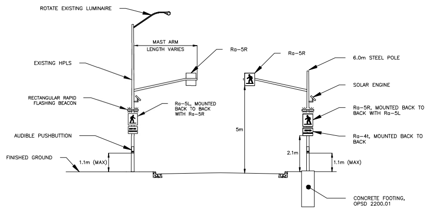
POLE INSTALLATION TYPE B N.T.S.
